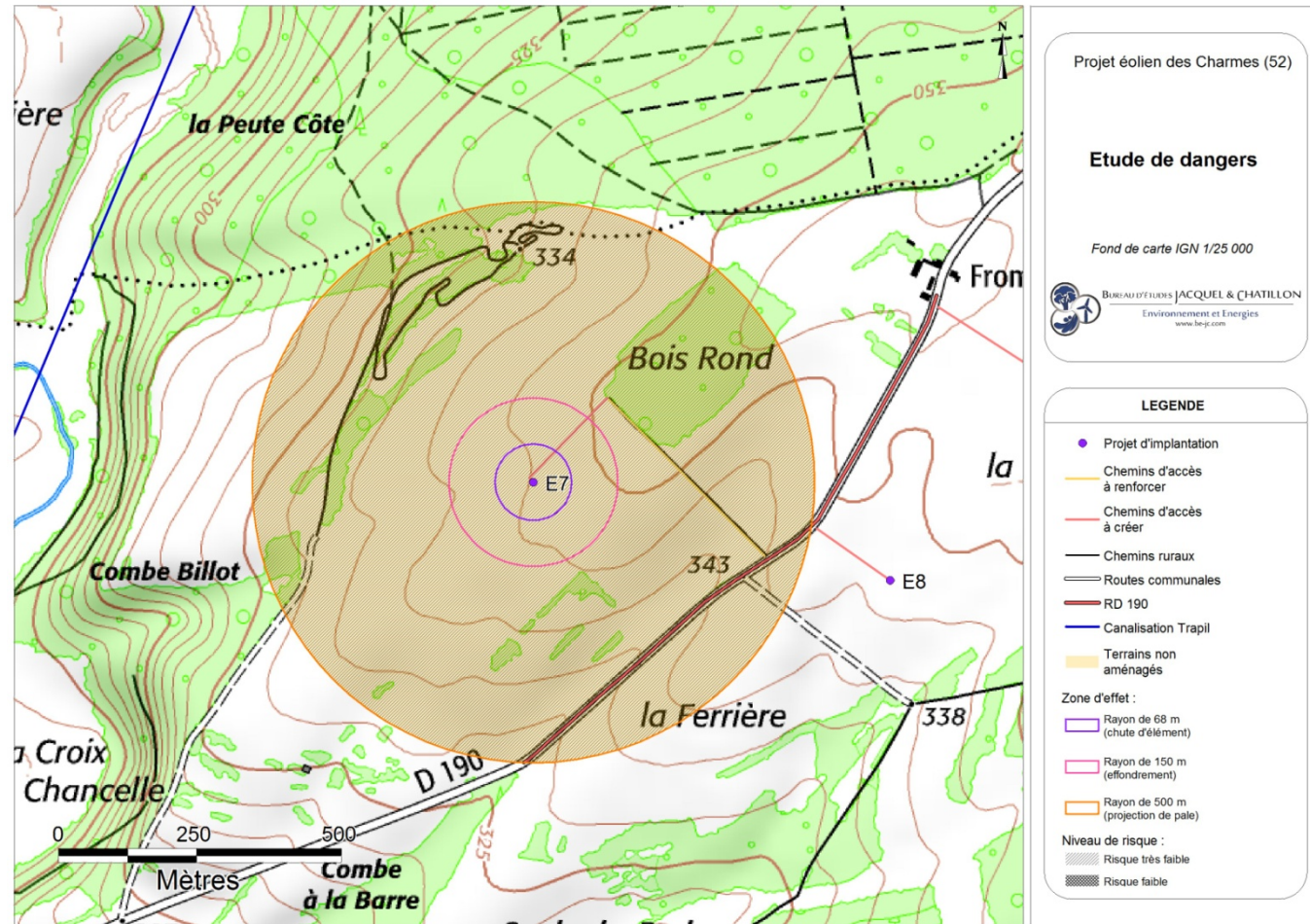
Carte 31 : Éolienne n°7 – Risques liés à l'effondrement de l'éolienne, à la chute d'élément de l'éolienne, et à la projection de pale ou de fragment de pale (Source : BE Jacquel et Chatillon)
