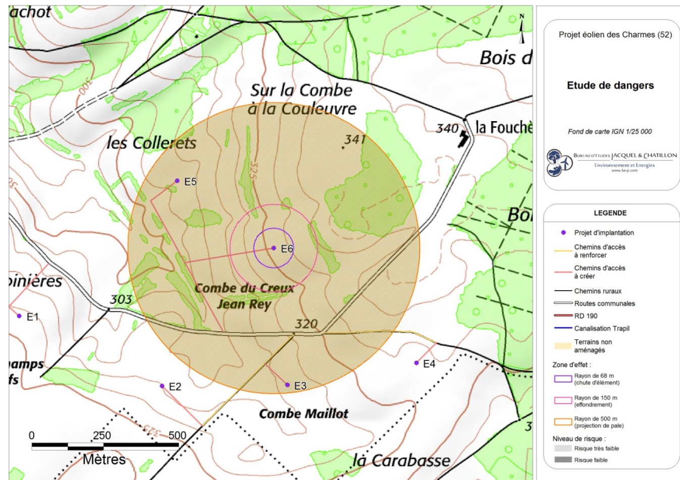
Carte 29 : Éolienne n°6 – Risques liés à l'effondrement de l'éolienne, à la chute d'élément de l'éolienne, et à la projection de pale ou de fragment de pale (Source : BE Jacquel et Chatillon)
