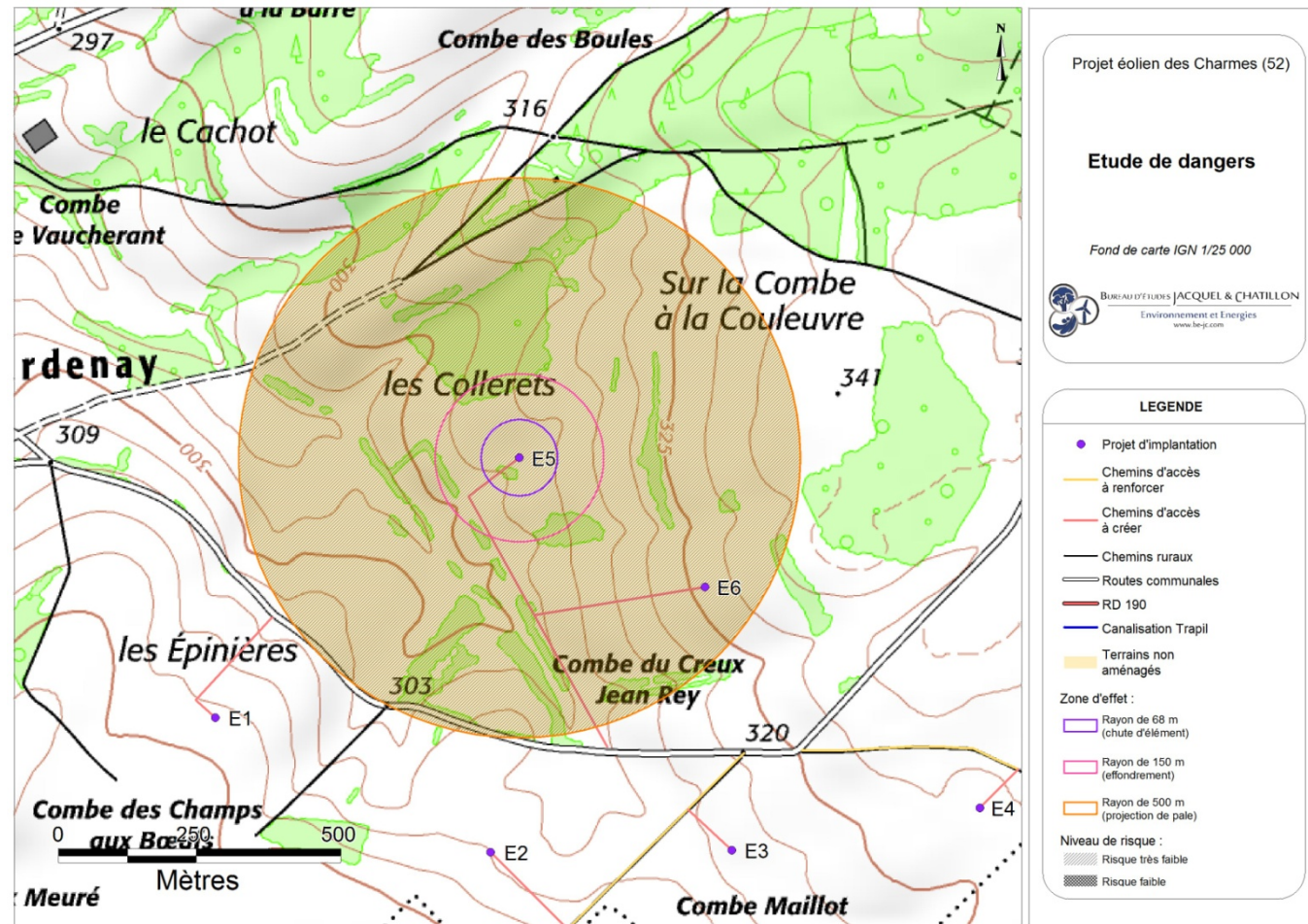
Carte 27 : Éolienne n°5 – Risques liés à l'effondrement de l'éolienne, à la chute d'élément de l'éolienne, et à la projection de pale ou de fragment de pale (Source : BE Jacquel et Chatillon)
