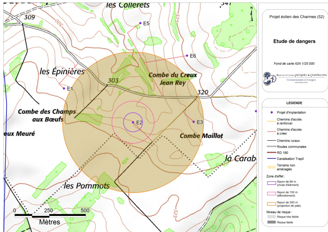
Carte 21 : Éolienne n°2 – Risques liés à l'effondrement de l'éolienne, à la chute d'élément de l'éolienne, et à la projection de pale ou de fragment de pale (Source : BE Jacquel et Chatillon)
