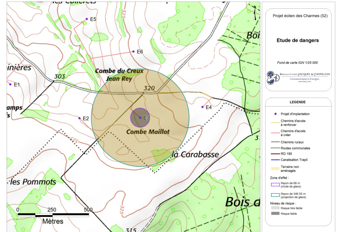
Carte 24 : Éolienne n°3 – Risques liés à la chute et à la projection de glace (Source : BE Jacquel et Chatillon)
