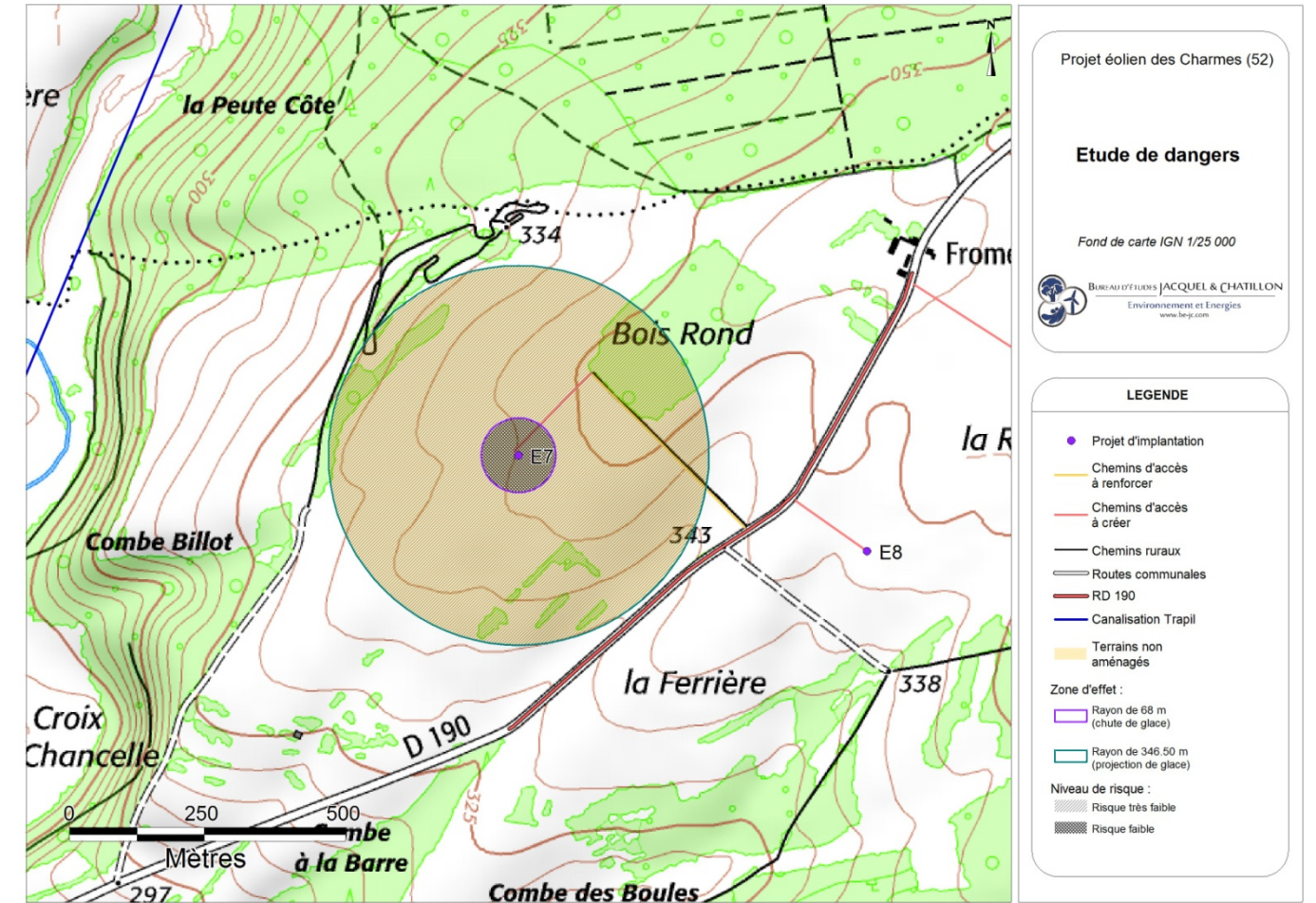
Carte 32 : Éolienne n°7 – Risques liés à la chute et à la projection de glace (Source : BE Jacquel et Chatillon)
