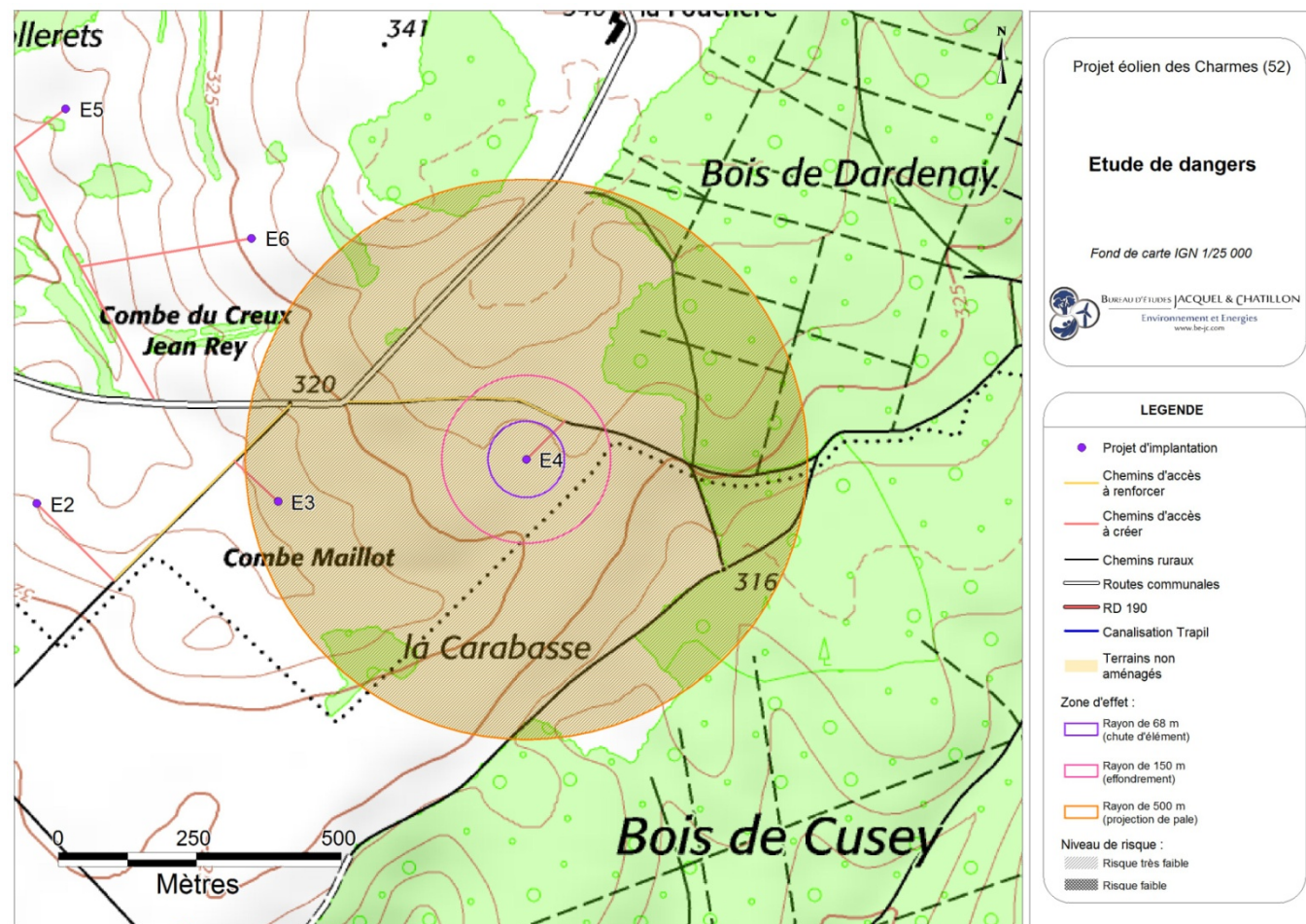
Carte 25 : Éolienne n°4 – Risques liés à l'effondrement de l'éolienne, à la chute d'élément de l'éolienne, et à la projection de pale ou de fragment de pale (Source : BE Jacquel et Chatillon)
