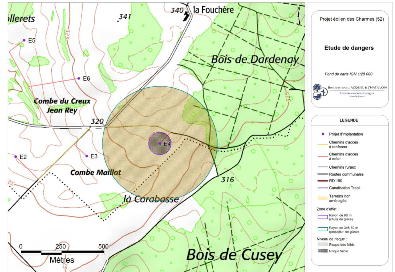
Carte 26 : Éolienne n°4 – Risques liés à la chute et à la projection de glace (Source : BE Jacquel et Chatillon)
