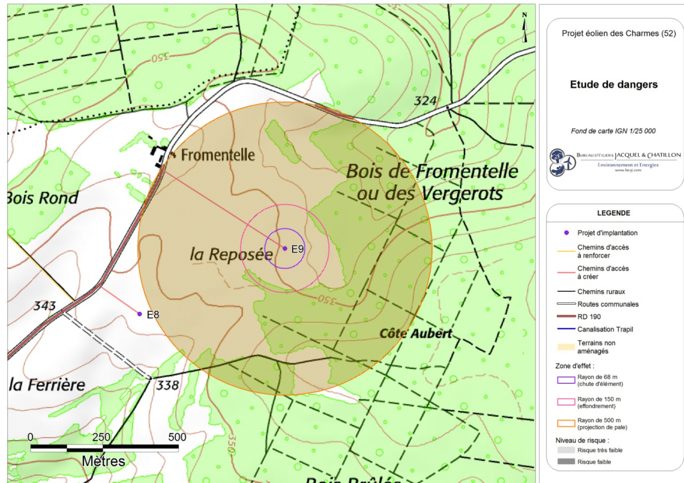
Carte 35 : Éolienne n°9 – Risques liés à l'effondrement de l'éolienne, à la chute d'élément de l'éolienne, et à la projection de pale ou de fragment de pale (Source : BE Jacquel et Chatillon)
