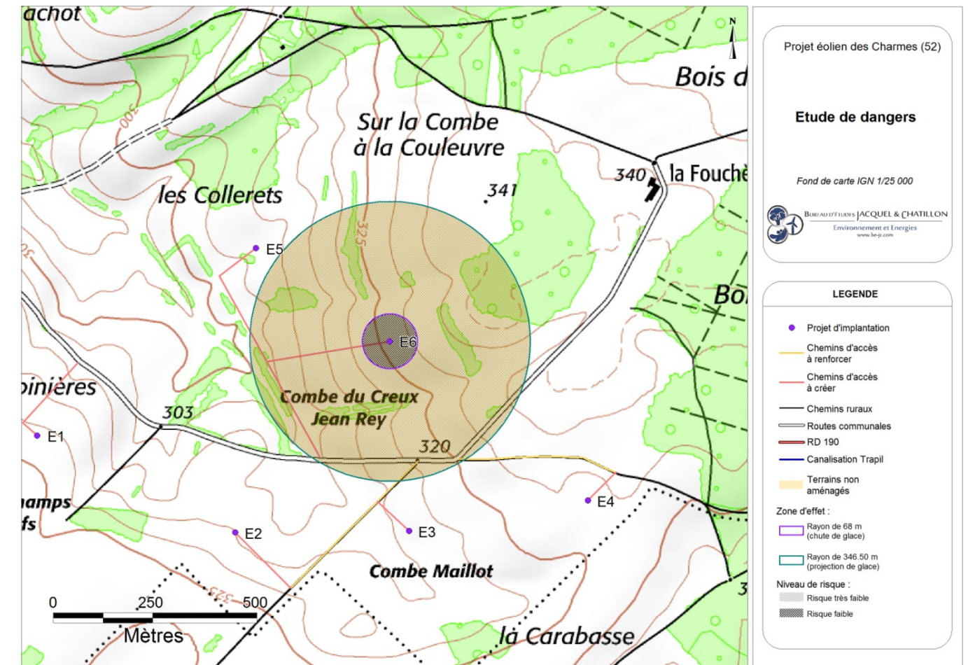
Carte 30 : Éolienne n°6 – Risques liés à la chute et à la projection de glace (Source : BE Jacquel et Chatillon)
