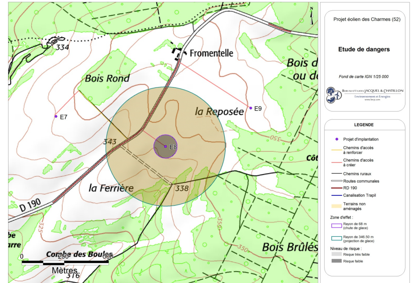
Carte 34 : Éolienne n°8 – Risques liés à la chute et à la projection de glace (Source : BE Jacquel et Chatillon)
