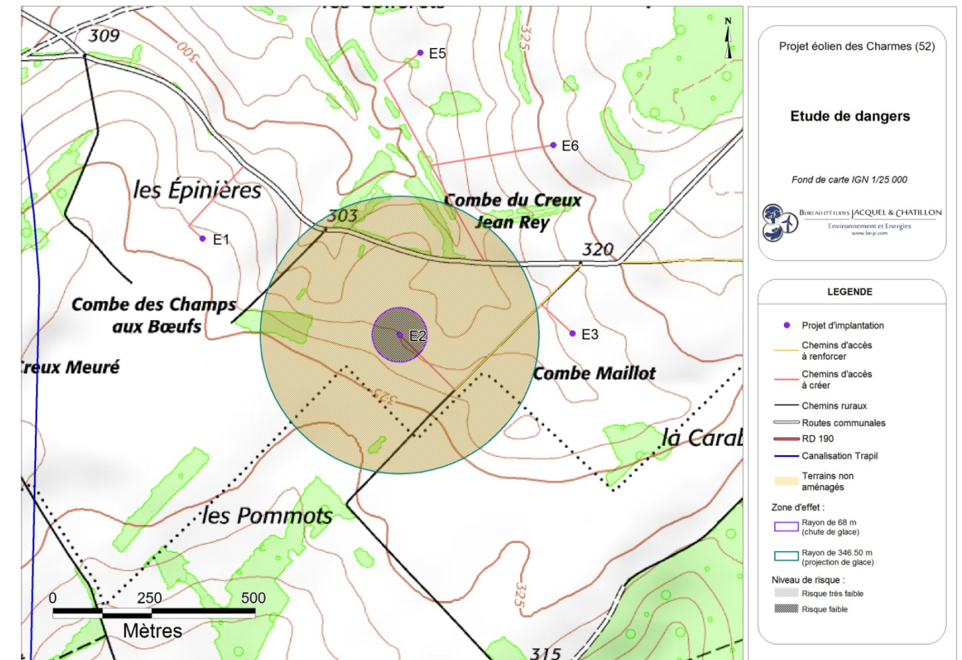
Carte 22 : Éolienne n°2 – Risques liés à la chute et à la projection de glace (Source : BE Jacquel et Chatillon)
