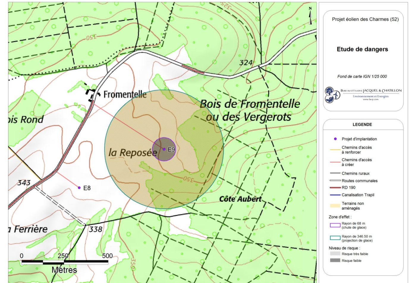
Carte 36 : Éolienne n°9 – Risques liés à la chute et à la projection de glace (Source : BE Jacquel et Chatillon)
