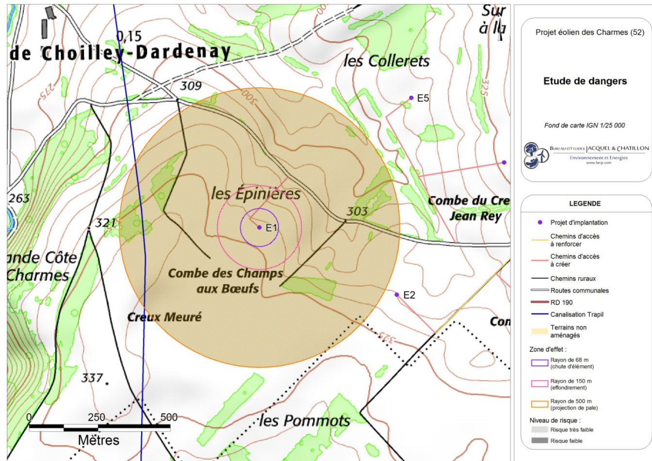
Carte 19 : Éolienne n°1 – Risques liés à l'effondrement de l'éolienne, à la chute d'élément de l'éolienne, et à la projection de pale ou de fragment de pale (Source : BE Jacquel et Chatillon)
