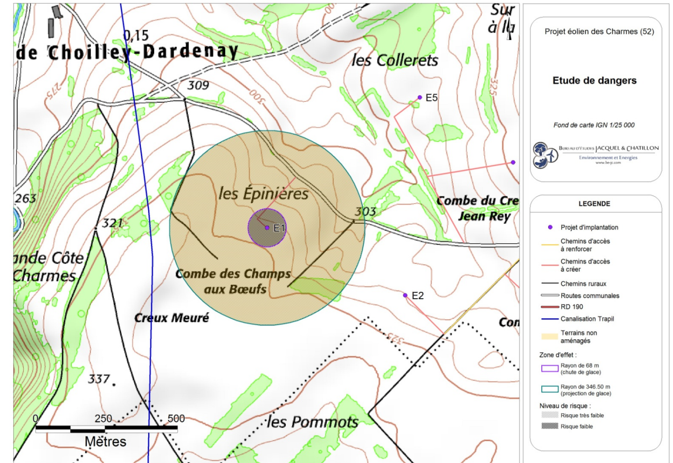
Carte 20 : Éolienne n°1 – Risques liés à la chute et à la projection de glace (Source : BE Jacquel et Chatillon)
