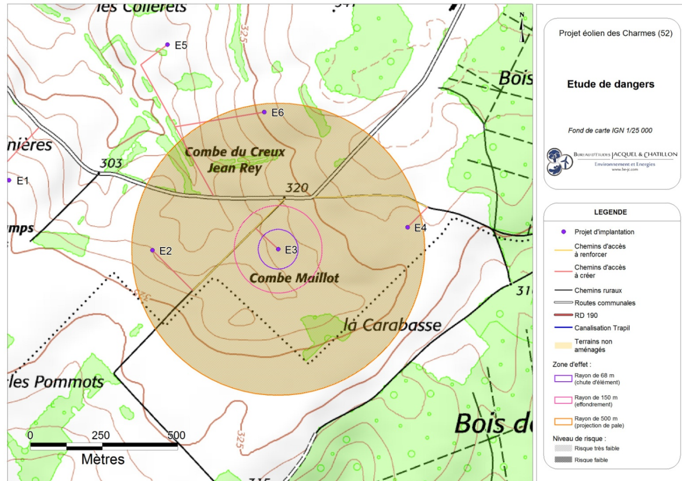
Carte 23 : Éolienne n°3 – Risques liés à l'effondrement de l'éolienne, à la chute d'élément de l'éolienne, et à la projection de pale ou de fragment de pale (Source : BE Jacquel et Chatillon)
