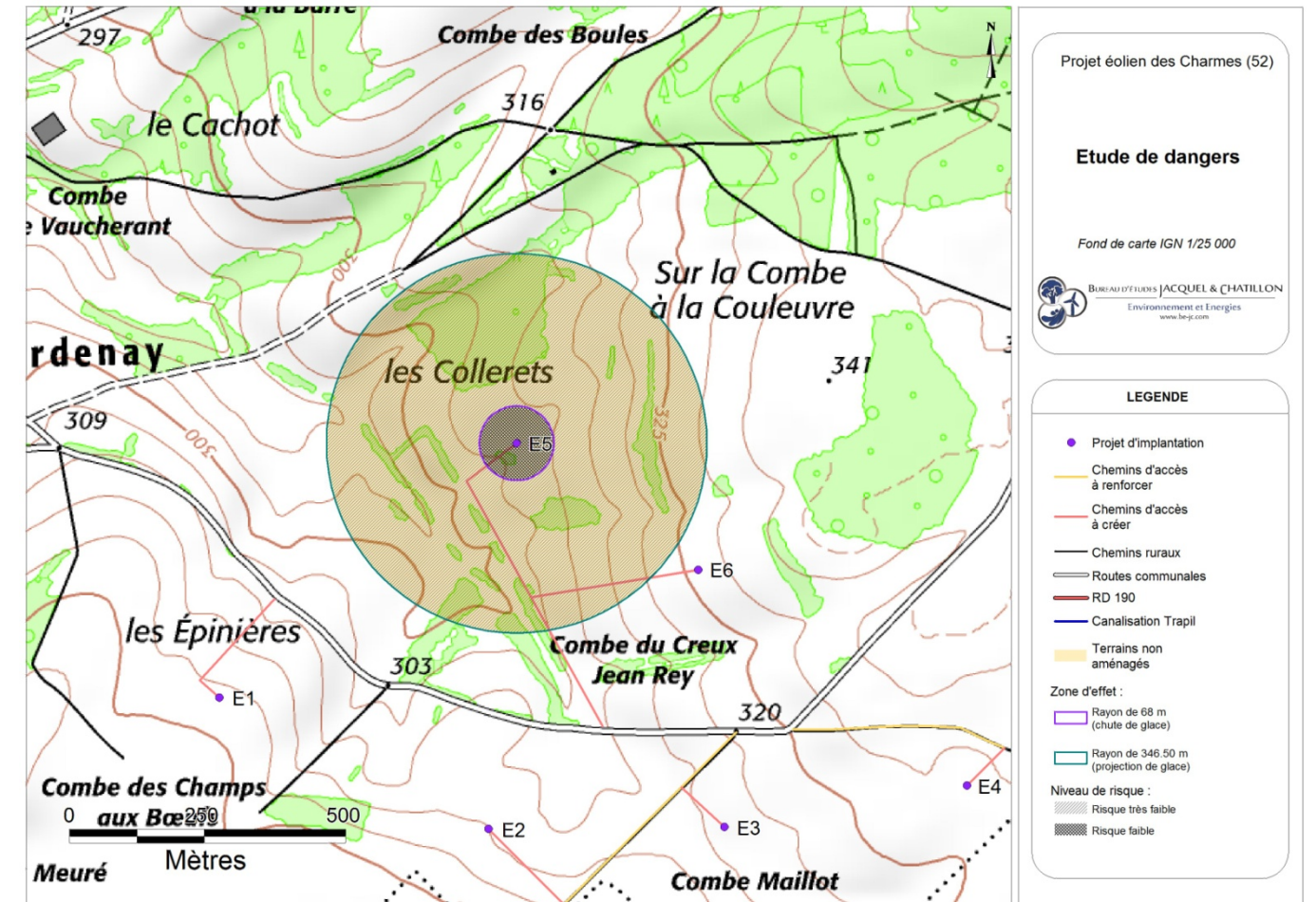
Carte 28 : Éolienne n°5 – Risques liés à la chute et à la projection de glace (Source : BE Jacquel et Chatillon)
