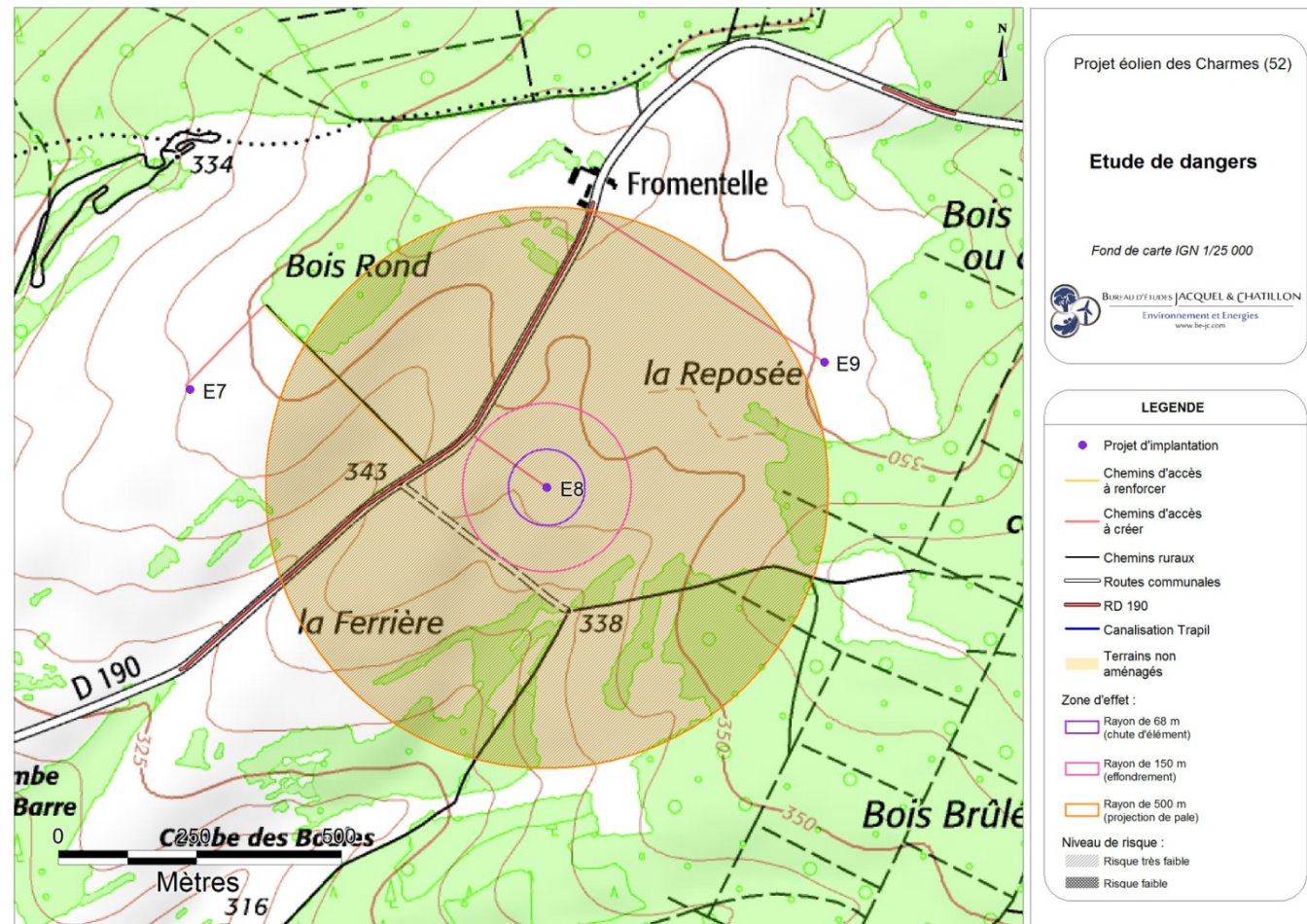
Carte 33 : Éolienne n°8 – Risques liés à l'effondrement de l'éolienne, à la chute d'élément de l'éolienne, et à la projection de pale ou de fragment de pale (Source : BE Jacquel et Chatillon)
